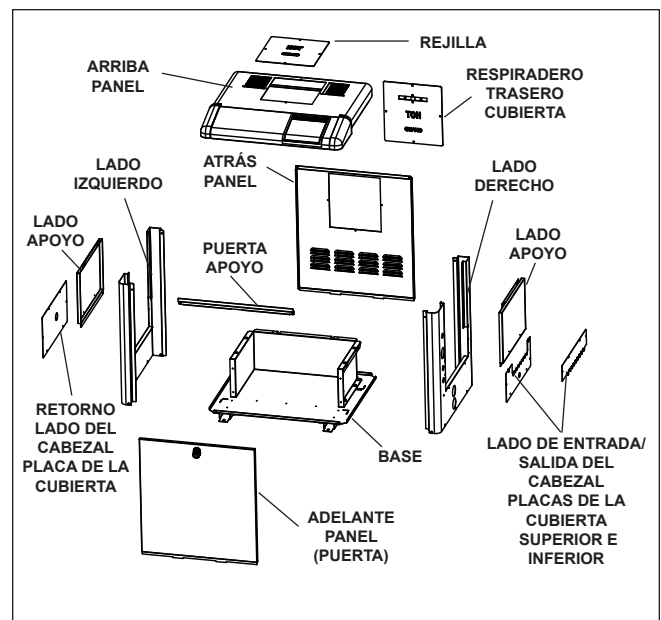
Figura 13. Identificación del panel del LXi
