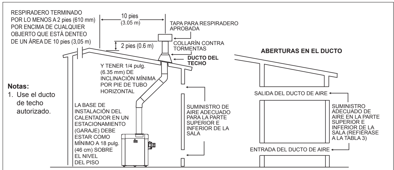
Figura 7. Ventilación instalada en interiores (EEUU) o en exteriores con protección (Canadá)
