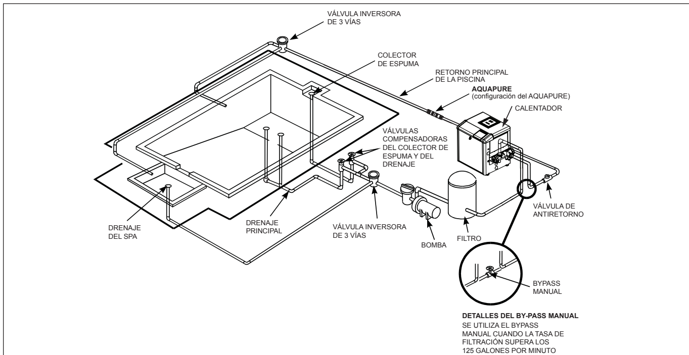
Figura 10. Instalación típica de tubería
