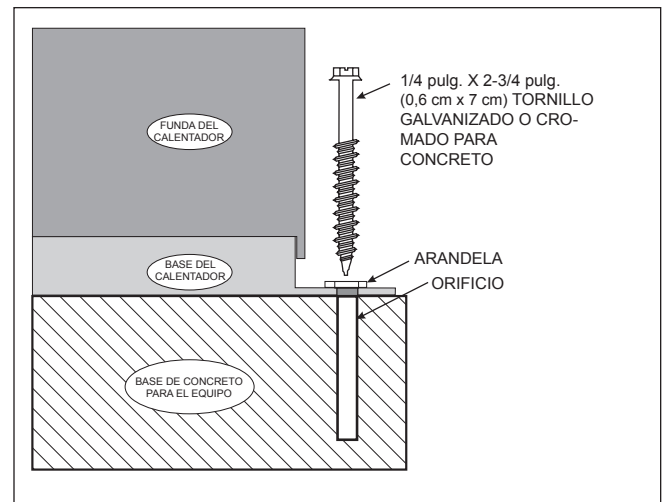
Figura 4. Instale el calentador en la plataforma del equipo
