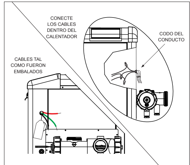
Figura 21. Conexiones del cableado en terreno
