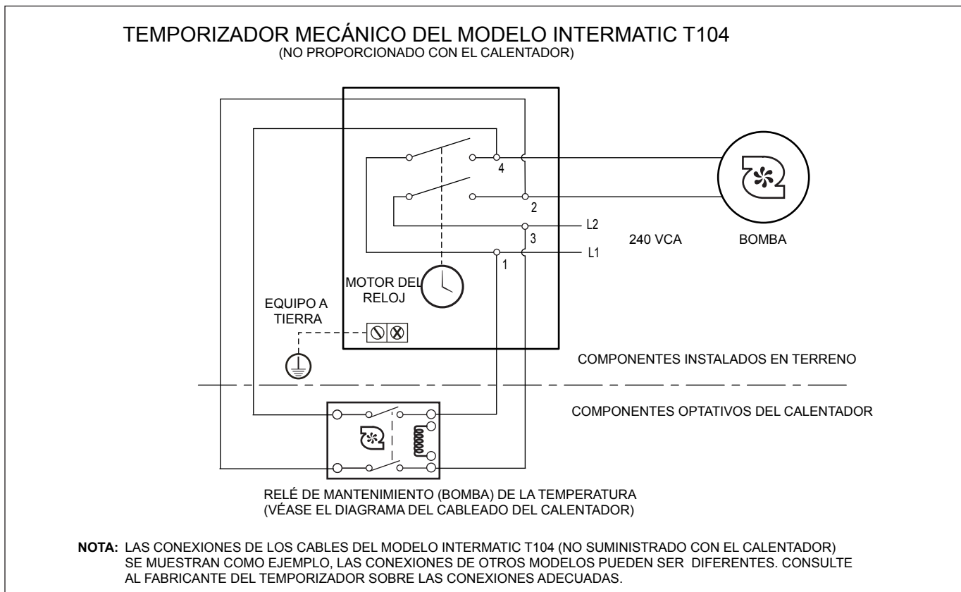
Figura 24. Ejemplo del cableado del mantenimiento de la temperatura hacia el reloj
