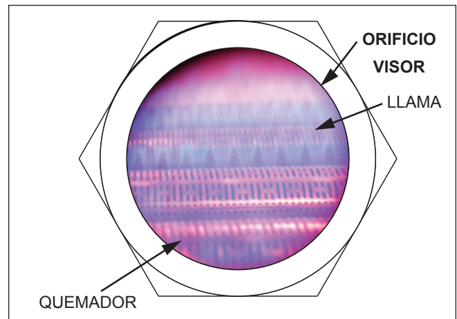
Figura 36. Vista de la llama
