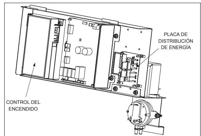
Figura 22. Ubicación de la placa de distribución de energía
