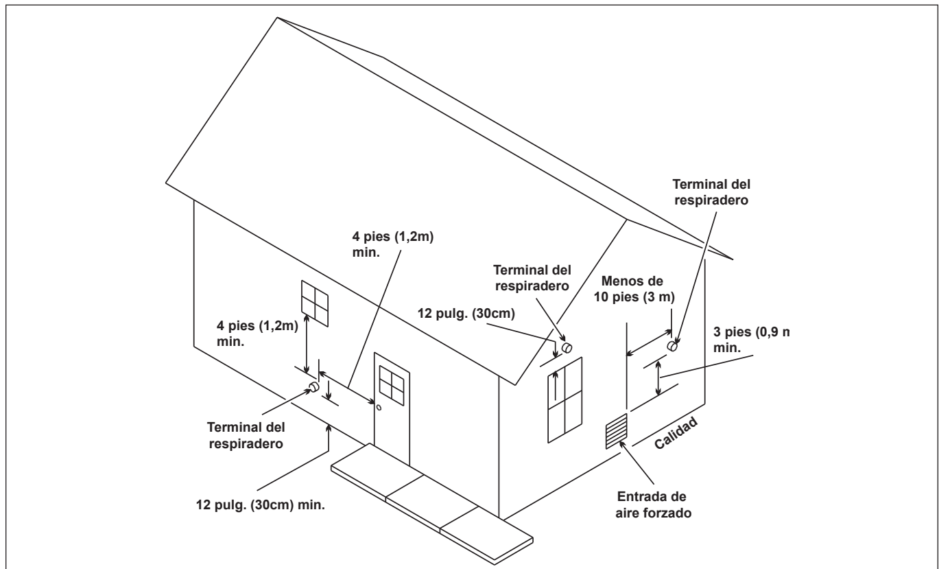
Figura 8. Terminales de ventilación de paredes laterales
